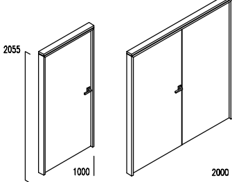
Puerta ciega E50 Solid doors T50 Porte pleine E50
