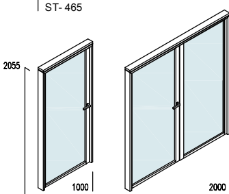
Puerta mono-vidrio enmarcado E50 ( 6+6 ó 5+5 mm ) Framed single glass door T50 (5+5 or 6+6 mm) Porte simple verre encadré E50 ( 6+6 ou 5+5 mm )
