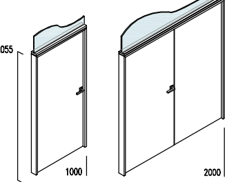
INSERTO EN ST-100 INSERTED INTO ST-100 INSERE EN ST-100
