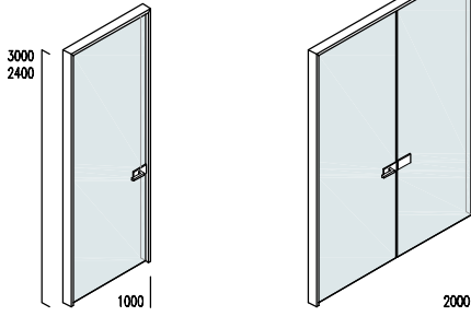
Puerta mono-vidrio enmarcado E50 ( 6+6 ó 5+5 mm ) Framed single glass door T50 (5+5 or 6+6 mm) Porte simple verre encadré E50 ( 6+6 ou 5+5 mm )
