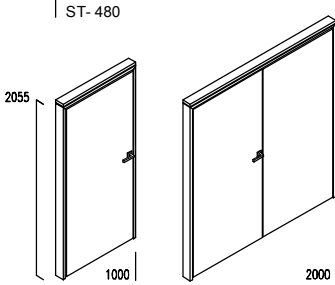
Puerta ciega E100 Solid doors T100 Porte pleine E100
