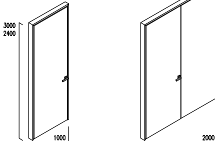
Puerta ciega E100 Solid doors T100 Porte pleine E100
